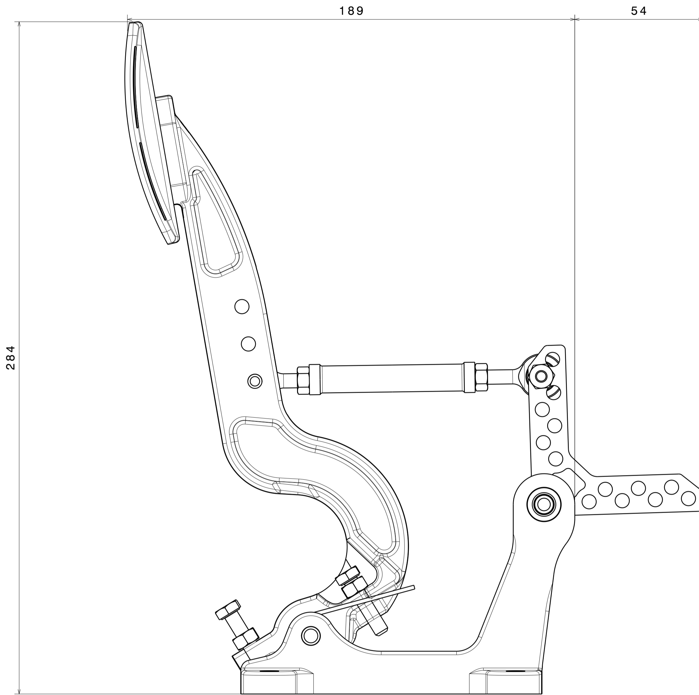
Front view Scale: 1:1
